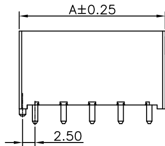
2x02P~2x06P 视图
