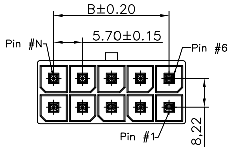
2x02P~2x06P 视图
