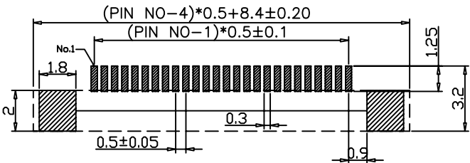
适用线路板 RECOMMENDED PCB LAYOUT
