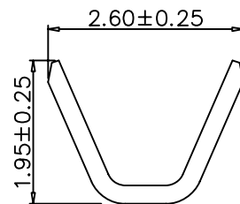
A-A
