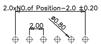
P.C.B LAYOUT
