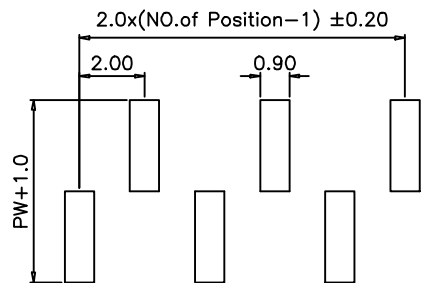
P.C.B LAYOUT A Type
