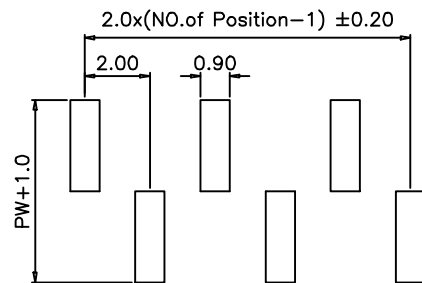
P.C.B LAYOUT B Type
