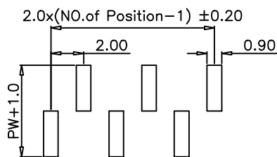
P.C.B LAYOUT A Type
