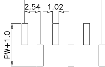
P.C.B LAYOUT B Type
