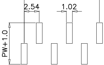
P.C.B LAYOUT A Type
