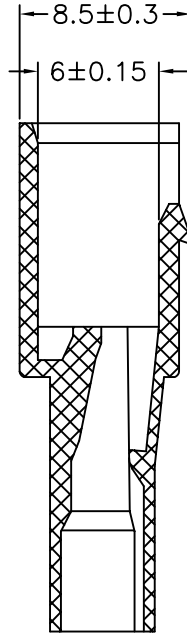
SEC:A-A
