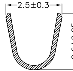
SEC:A-A
