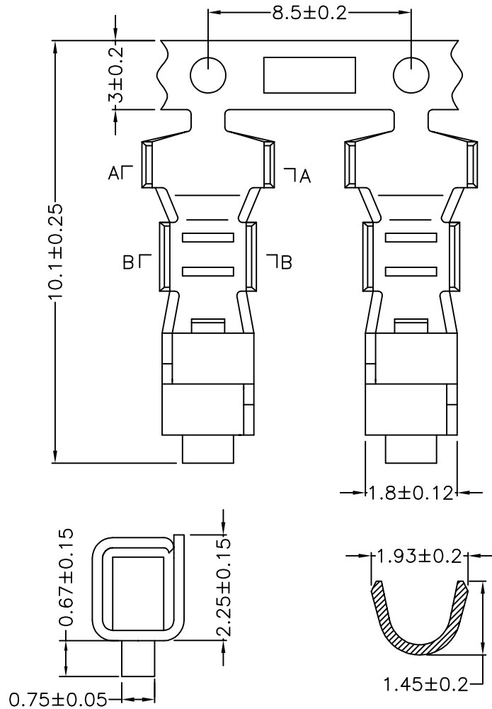
SEC:B-B
